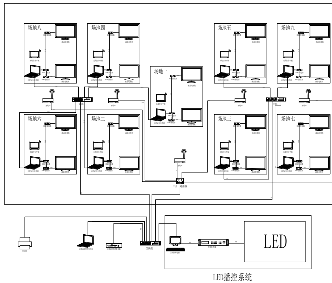
乒乓球比赛记分系统
